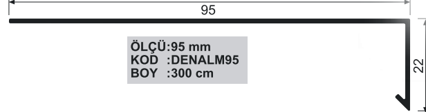
95 mm Alüminyum Denizlik
