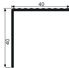
40X40 MERDİVEN KÖŞEBENTİ
