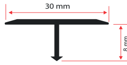
30 mm Parlak Alm.T Profil
