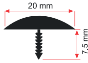
20 mm Alüminyum Bombeli T Profili
