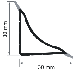
PVC YUMUŞAKSIZ KÜVET KENAR PROFİLİ PVC BATHTUBE EDGE PROFILE ( SOLID ) ПВХ ПРОФИЛЬ БЕЗ РЕЗИНОЙ КРАЕВ ВАНН
