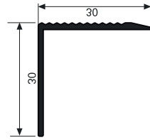
30X30 MERDİVEN KÖŞEBENTİ
