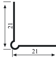
PVC KESİK ALÇI KÖŞE PROFİLLERİ (Kemer Profili)
