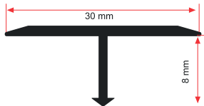
30 mm Alüminyum T Profili
