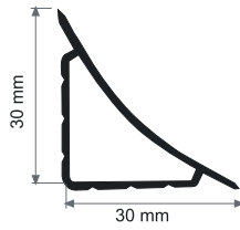
PVC YUMUŞAKSIZ KÜVET KENAR PROFİLİ PVC BATHTUBE EDGE PROFILE ( SOLID ) ПВХ ПРОФИЛЬ БЕЗ РЕЗИНОЙ КРАЕВ ВАНН
