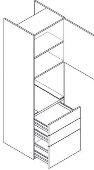
ÜNİTE KODU: 7060D24 ÜNİTE ADI: 60x216x56 Cm Ankastre Fırın Boy Dolabı
