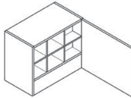
ÜNİTE KODU: 7060A23 ÜNİTE ADI: 60x50x33 Cm Sürgülü Aspiratör Dolap
