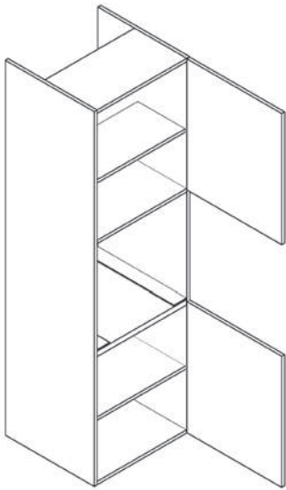
ÜNİTE KODU: 7060D26 ÜNİTE ADI: 60x216x56 Cm Ank. Fırın Boy Dolabı
