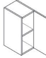
ÜNİTE KODU: 7025A21 ÜNİTE ADI: 25x72x33 Cm Asma Dolap
