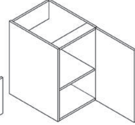
ÜNİTE KODU: 7045B01 ÜNİTE ADI: 45x84x56 Cm Alt Dolap
