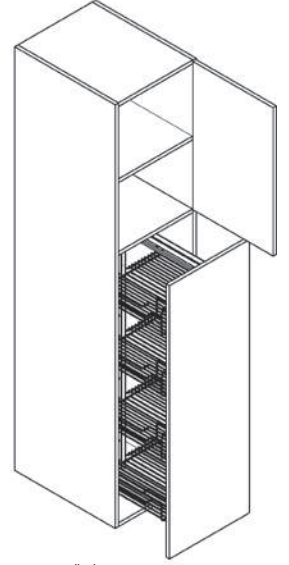
ÜNİTE KODU: 7045C22 ÜNİTE ADI: 45x216x56 Cm Kiler Dolabı
