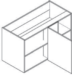
ÜNİTE KODU: 70120B31 ÜNİTE ADI: 120x84x56 Cm Alt Köşe Dolabı (Rafli)
