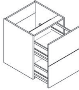
ÜNİTE KODU: 7060B02 ÜNİTE ADI: 60x84x56 Cm İki Çekmeceli Alt Dolap
