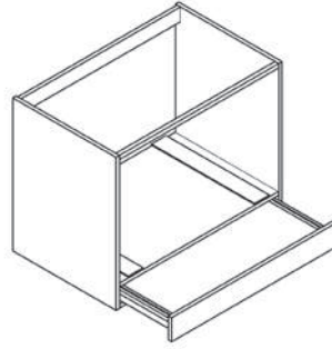
ÜNİTE KODU: 7090B10 ÜNİTE ADI: 90x84x56 Cm Ankastr Fırın Dolabı
