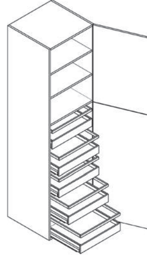
ÜNİTE KODU: 7060C36 ÜNİTE ADI: 60x240x56 Cm Serbest Sepetli Boy Kiler Dolabı (Plus Seri)
