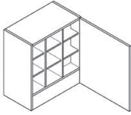
ÜNİTE KODU: 7060A33 ÜNİTE ADI: 60x68x33 Cm Sürgülü Aspiratör Dolap
