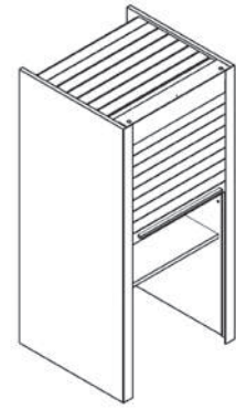
ÜNİTE KODU: 7060A57 ÜNİTE ADI: 60x128x56 Cm "Vetroline Cam"lı Stor Dolabı (Plus Seri)
