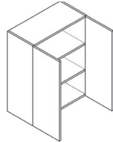
ÜNİTE KODU: 7070A31 ÜNİTE ADI: 70x90x33 Cm Asma Dolap
