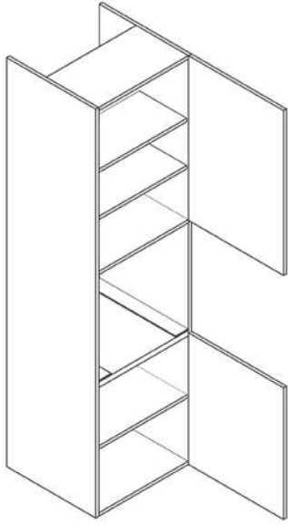
ÜNİTE KODU: 7060D36 ÜNİTE ADI: 60x234x56 Cm Ank. Fırın Boy Dolabı
