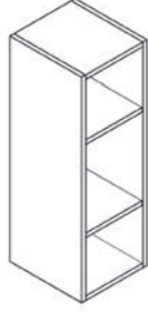
ÜNİTE KODU: 7030G31 ÜNİTE ADI: 30x90x33 Cm Açık Ünite (Renkli)
