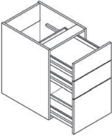
ÜNİTE KODU: 7045B03 ÜNİTE ADI: 45x84x56 Cm Üç Çekmeceli Alt Dolap
